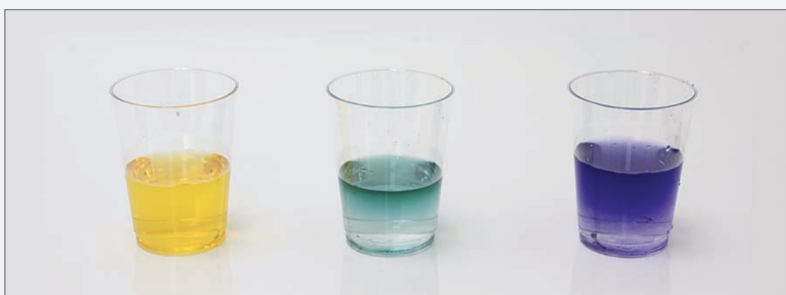
pH시약으로 pH농도 테스트를 해 본 결과 수돗물(사진 가운데)은 녹색의 약알칼리수(pH 8.0)로, 시중에서 유통되고 있는 생수(왼쪽)는 황색의 산성수(pH 5.5)로 나타났다. 이온수기를 통해 걸러낸 알칼리화원수(오른쪽)는 pH 9.0-9.5의 보라색 반응이 일어났다.
